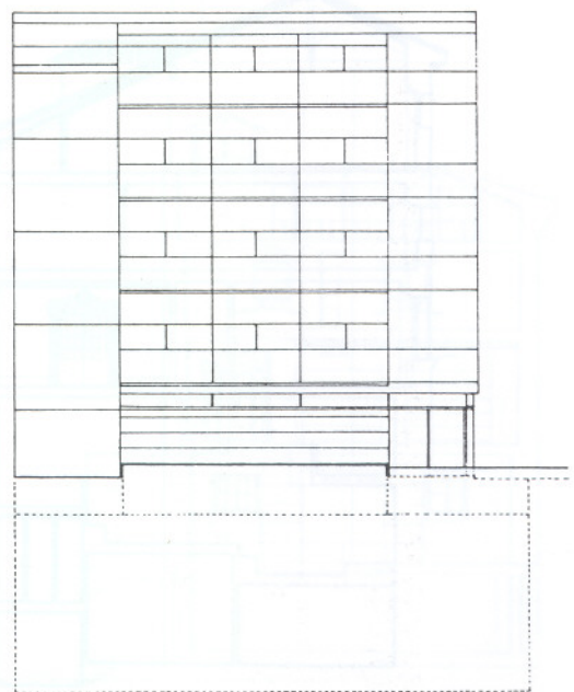
Alzado Posterior
