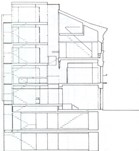
Sección Longitudinal
