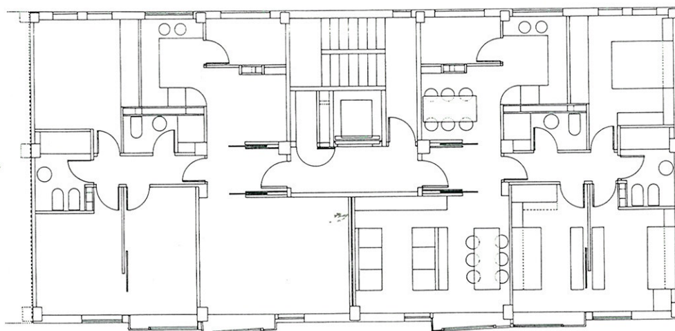
DETALLE PLANTA TIPO
