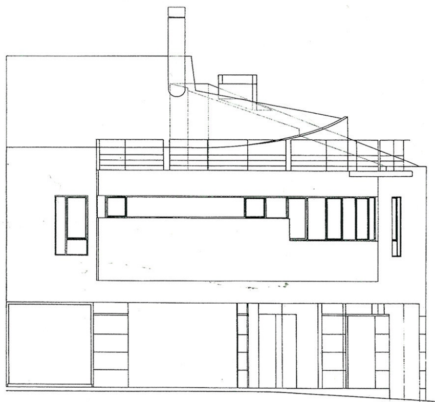
ALZADO NORTE
