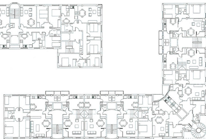
Planta tipo bloque 2
