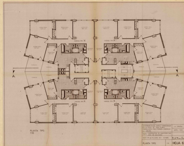
Anteproxecto do edificio “Torredorada” na rúa Juan Flórez. Planta tipo/ M a del Milagro Rey Hombre
